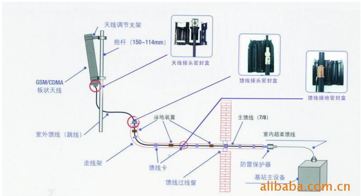
馈线接头的使用位置示意图。
